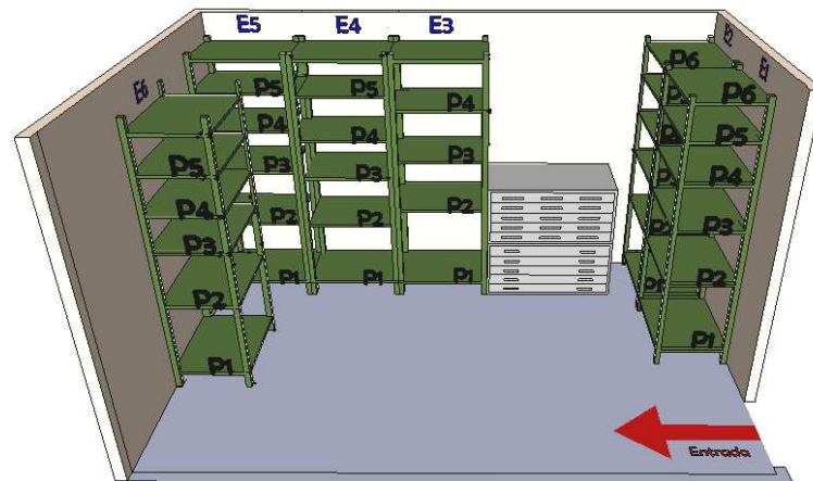
Fig.31. Mapeamento do sistema de localização existente. Modelo elaborado no software SketchUp Make®.
